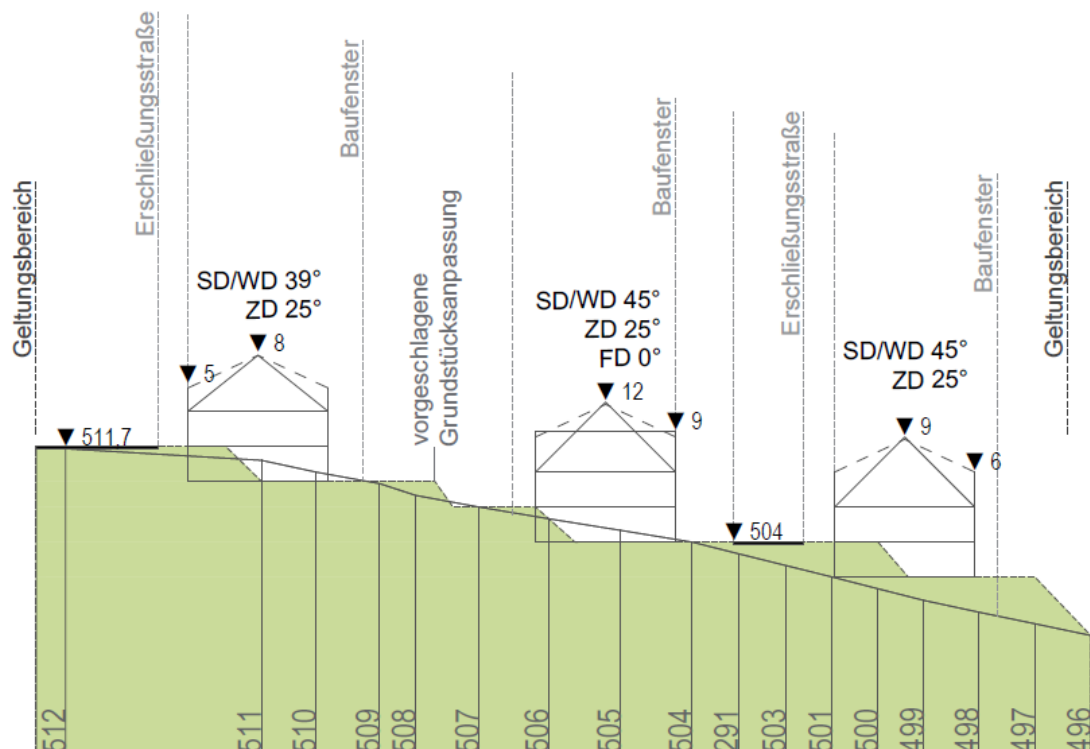
Schnitt B-B
